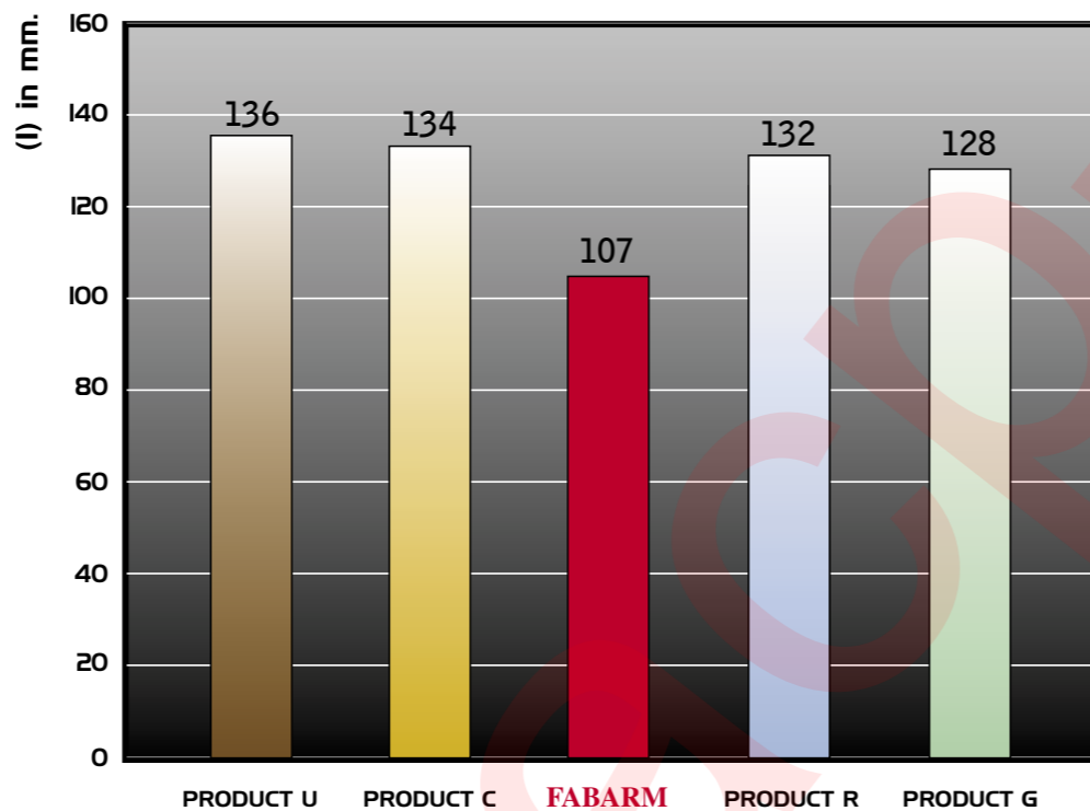
MUZZLE JUMP in mm ALZATA DELLA CANNA in mm RELEVEMENT DU CANON en mm ELEVACION DEL CAÑON en mm ELEVAÇÃO DO CANO em mm
